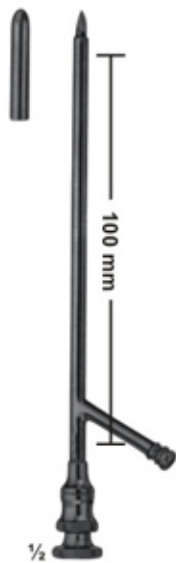
09-119 - 122 Inside diam Outside diam 09-119 3.0mm 40mm 09-120 3.6mm 4.6mm 09-121 4.3mm 5.3mm 09-122 6.0mm Gallbladder トロカール. OCHSNER
