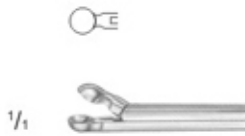
12-114 Hartmann-Herzfohl 20mm 'shaft 全長 '5mm
